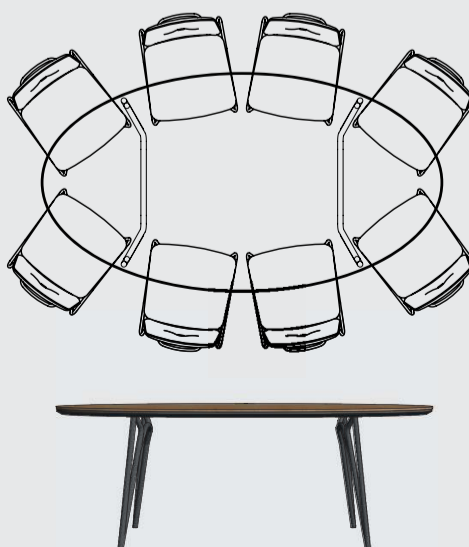
(Bar)tafel ovaal L220 x B120 x H77/92 CM Tafel art: 42099 Bartafel: 42401
