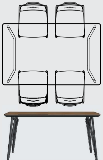
(Bar)tafel L160 x B100 x H77/92 CM Tafel art: 42093 Bartafel: 42398
